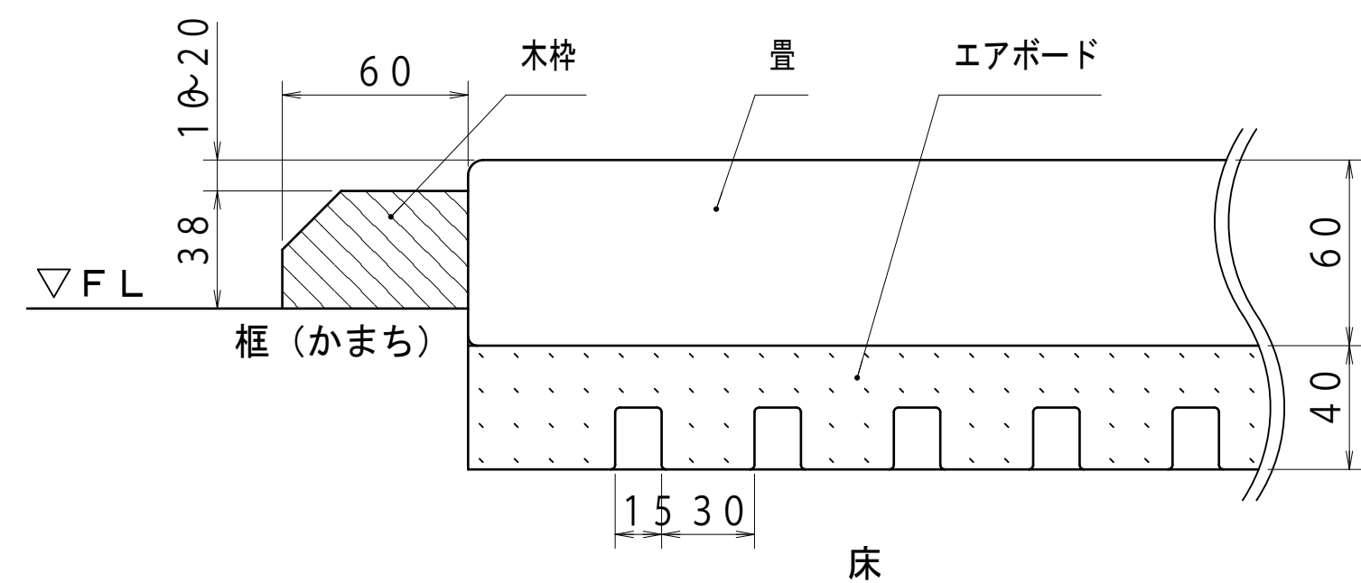
納まり断面図 S = 1 / 3
